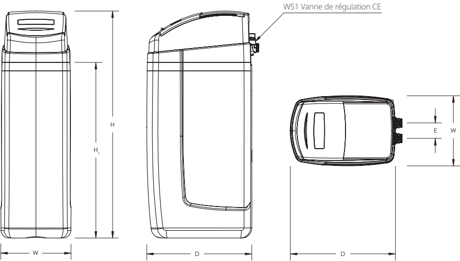
Dimensions des orifices de la vanne de régulation (hauteur d'orifice**, mm) Dimensions*, mm
