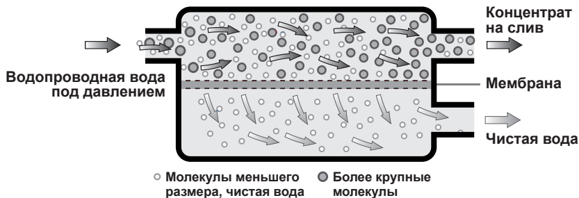
Рисунок 1. Обратный осмос
