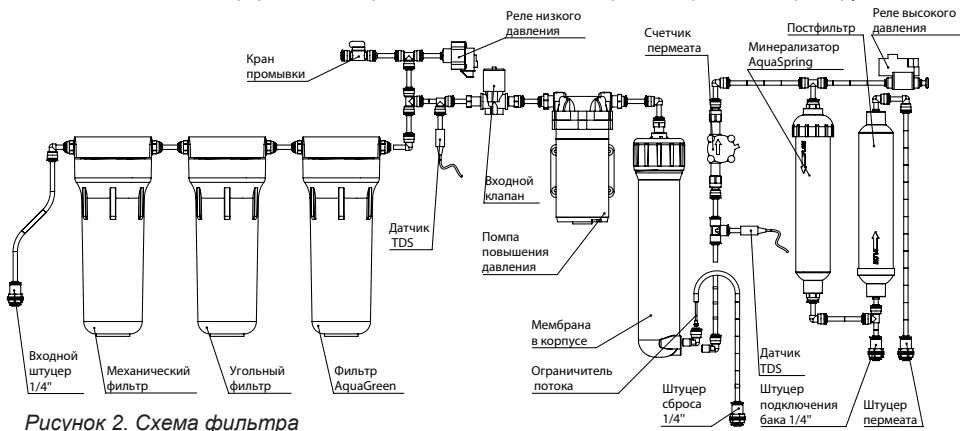
Рисунок 2. Схема фильтра
