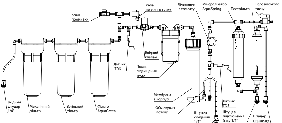
Рисунок 2. Схема фільтра
