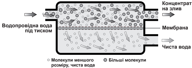
Рисунок 1. Зворотний осмос
